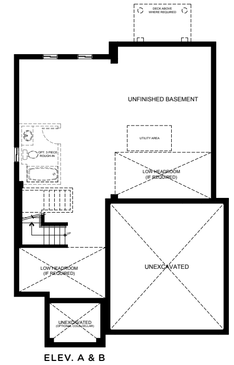
ELEV. A & B
