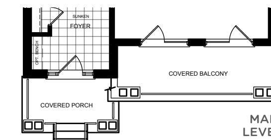
ELEV. C
