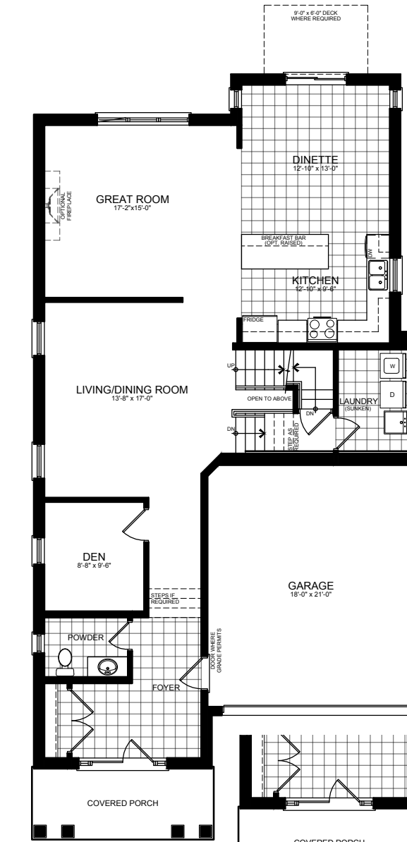
ELEV. A
