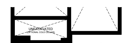
ELEV. C
