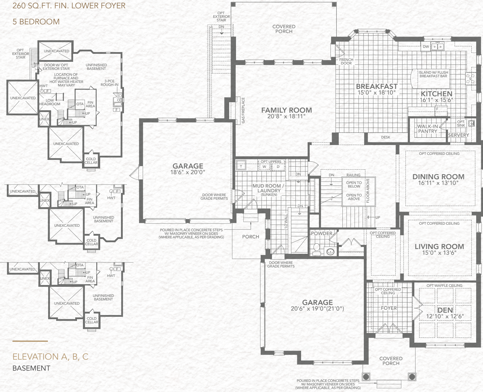
ELEVATION B
