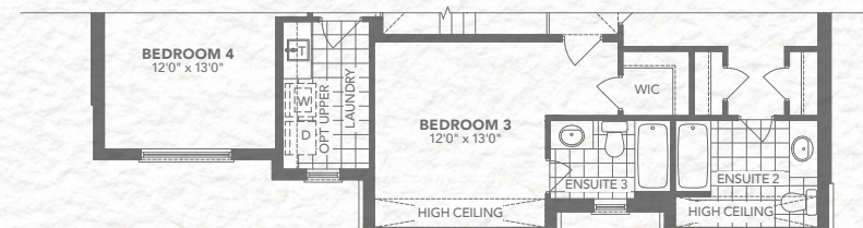
ELEVATION B
