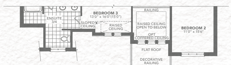
ELEVATION B
